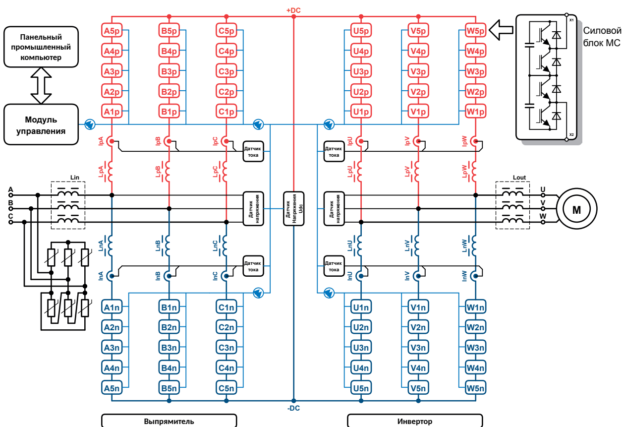
Функциональная схема силовой части преобразователя частоты ЭМСН
